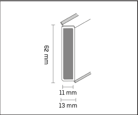
Tehnicka slika, presjek Cubu Decor
