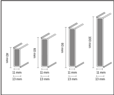
Tehnicka slika, presjek Cubu Flex
