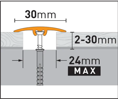
Presjek lajsne SM1
