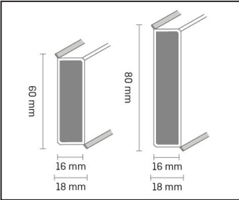
Tehnicka slika, presjek Cubu Flex life XL
