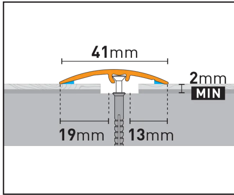
Presjek lajsne SM2
