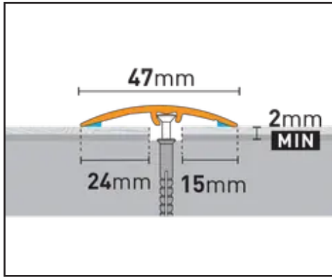
Presjek lajsne SM3
