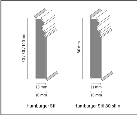
Tehnicka slika, presjek Cubu Hamburger
